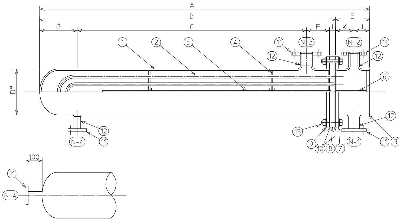
縦方向ニ設置スル場合 ノズルN-4取付位置詳細
