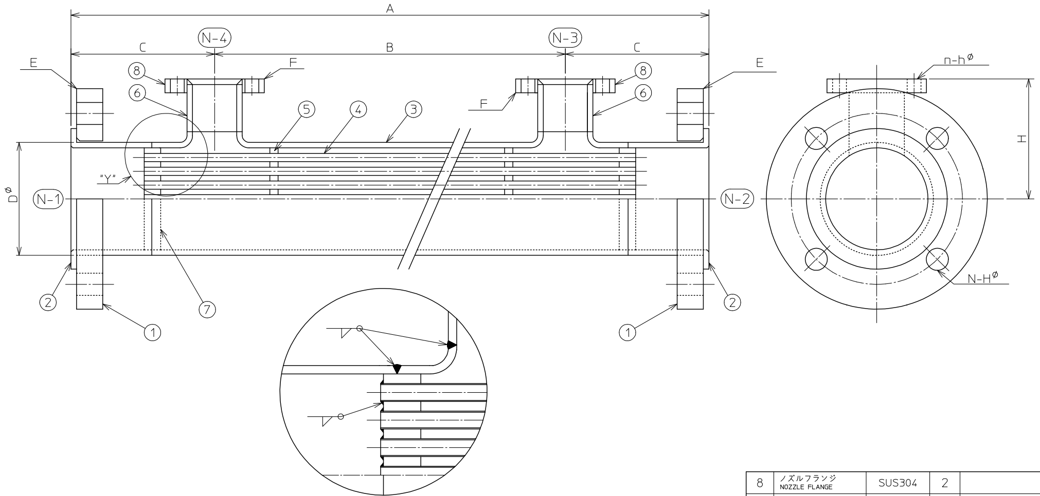
"Y" 部詳細 detail Y
