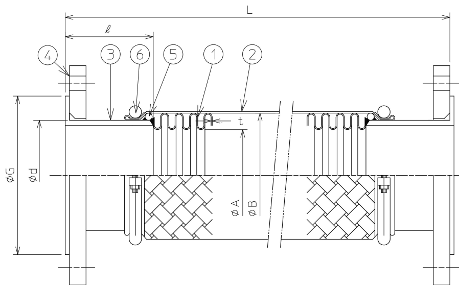
図1. 構造
